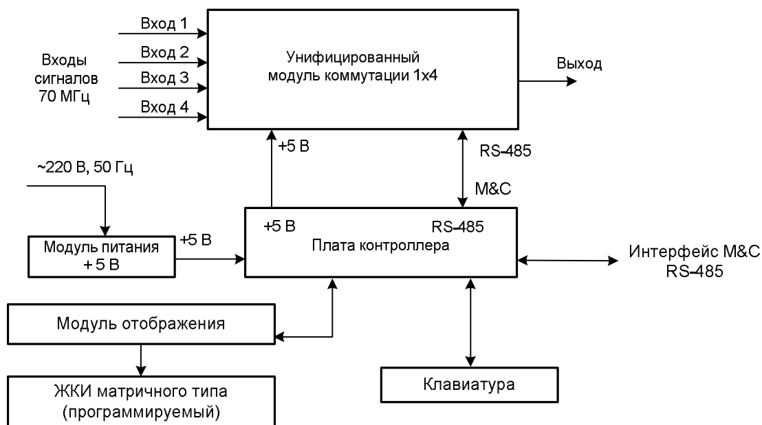
Рисунок 1.2 - Функциональная схема коммутатора 1x4 70 МГц
